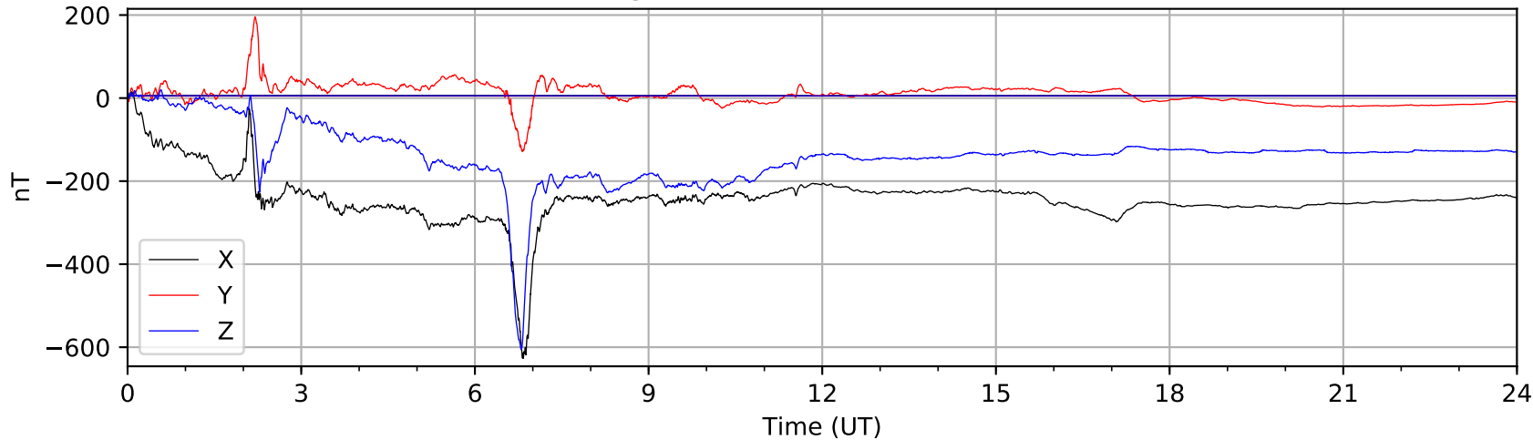
Bartington MAG03 (AUGO) 2021-08-28
