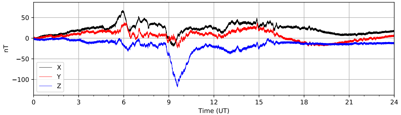
Bartington MAG03 (AUGO) 2020-11-29
