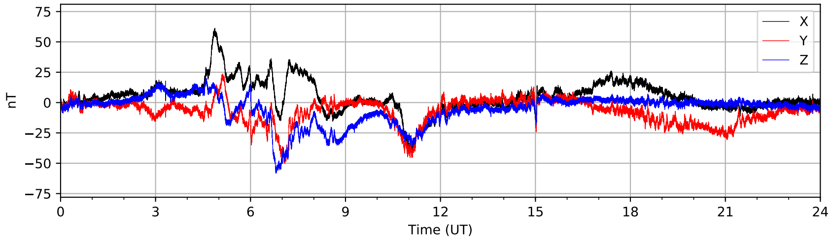
Bartington MAG03 (AUGO) 2020-11-23
