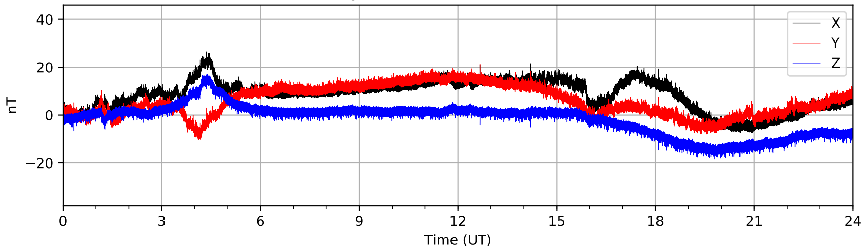
Bartington MAG03 (AUGO) 2020-11-15
