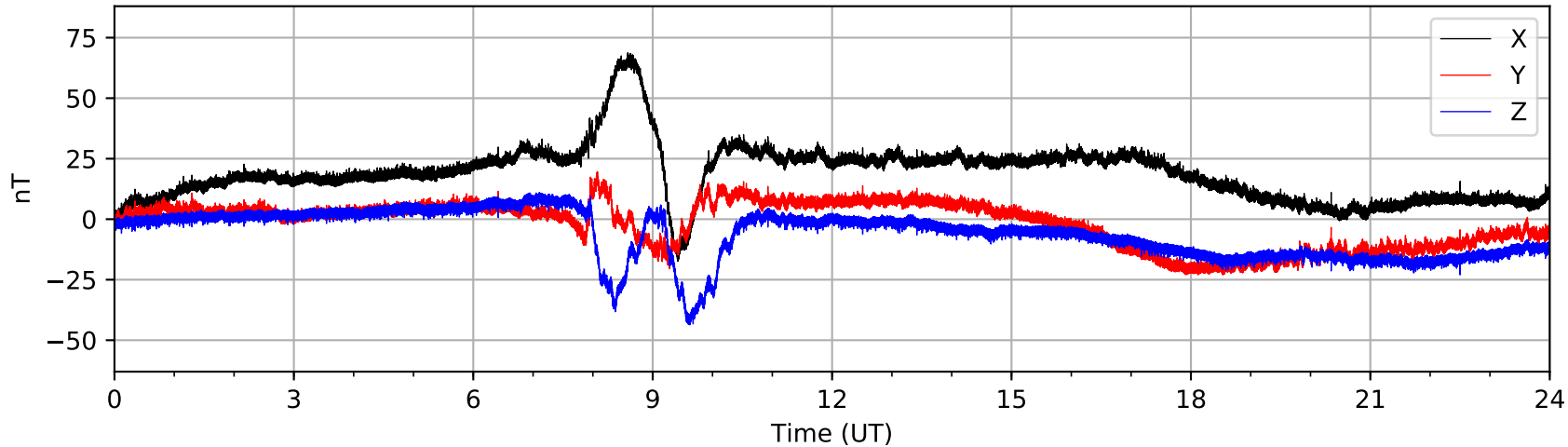
Bartington MAG03 (AUGO) 2020-11-12
