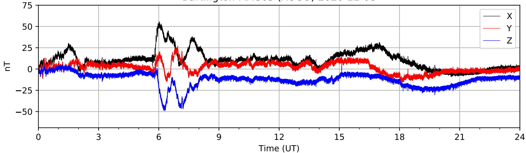
Bartington MAG03 (AUGO) 2020-11-08
